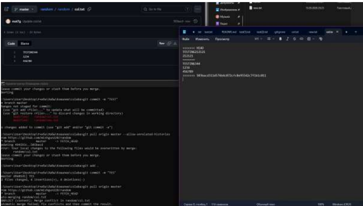
Рис. 31. - Получение конфликта слияния при совместной работе
